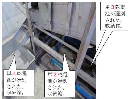
3. 廃棄乾電池類の大きさ選別機械
