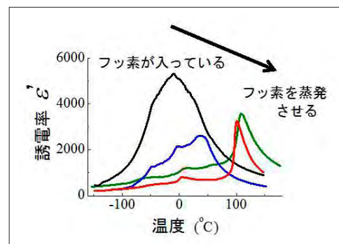
図4 フッ化カリウムで12%置換したチタン酸バリウム結晶における誘電率（電気を蓄えることが出来る量）の温度変化（結晶を高温でアニールすることで、山の位置が大きく変化している。）
