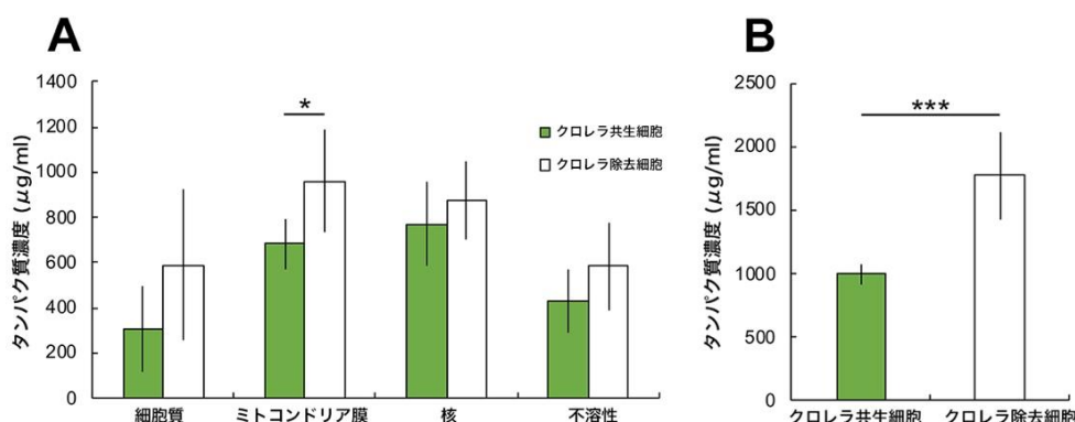
(図 5) (A) クロレラを除去したミドリゾウリムシおよびクロレラが共生しているミドリゾウリムシの 4 種類の細胞抽出液のタンパク質濃度。4 種類の抽出液は、細胞質・ミトコンドリア膜を含む膜・核・および不溶性タンパク質（細胞骨格）を含む。クロレラを除去したミドリゾウリムシのミトコンドリア膜タンパク質の濃度は、クロレラが共生しているミドリゾウリムシよりも高いことが分かる。(B) クロレラを除去したミドリゾウリムシおよびクロレラが共生しているミドリゾウリムシの細胞全体のタンパク質濃度を比較したグラフ。クロレラを除去したミドリゾウリムシのタンパク質濃度は、クロレラが共生しているミドリゾウリムシの約 1.8 倍であった。
